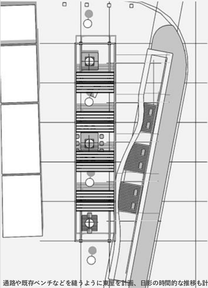
通路や既存ベンチなどを縫うように東屋を計画、日影の時間的な推移も計算して低予算で実現した
